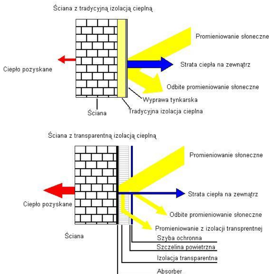
Rysunek 7. Przykład zastosowania izolacji transparentnej
