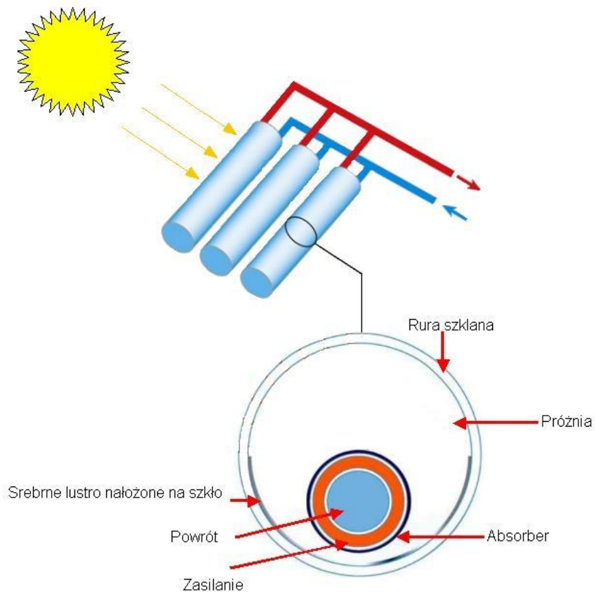
Rysunek 14. Budowa kolektora słonecznego próżniowo-rurowego
